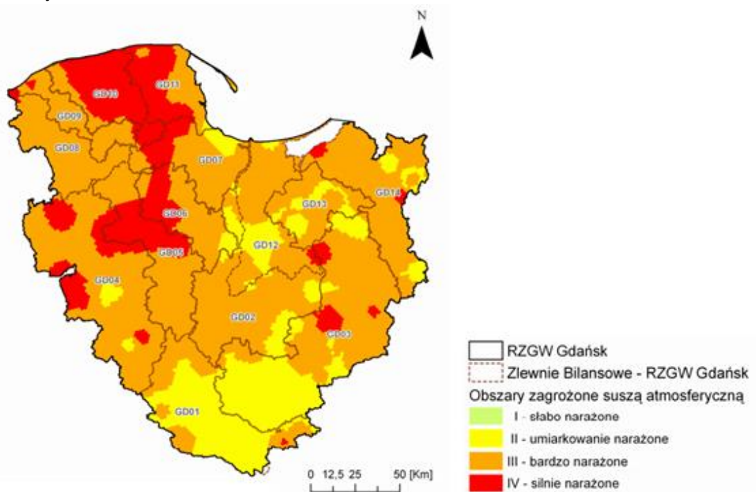
Rysunek 30. Obszary zagrożone suszą atmosferyczną na terenie RZGW w Gdańsku.
