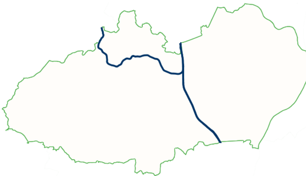
Rysunek 9. Układ linii kolejowych w powiecie gdańskim. źródło: PKP Polskie Linie Kolejowe S.A., opracowanie własne
