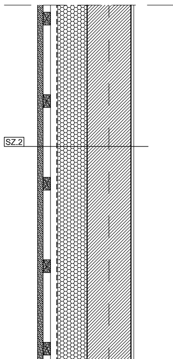
ŚCIANA Z ELEWACJĄ DREWNIANĄ przekrój pionowy
